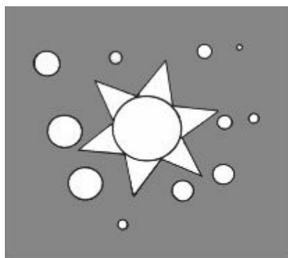
28. Le dessin représente notre système solaire, avec une planète supplémentaire.
