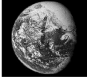
8. Photo satellite (Apollo 16) qui montre le trou.
