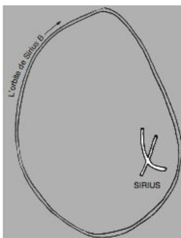
48. L'orbite de Sirius B d'après un dessin dogon.
